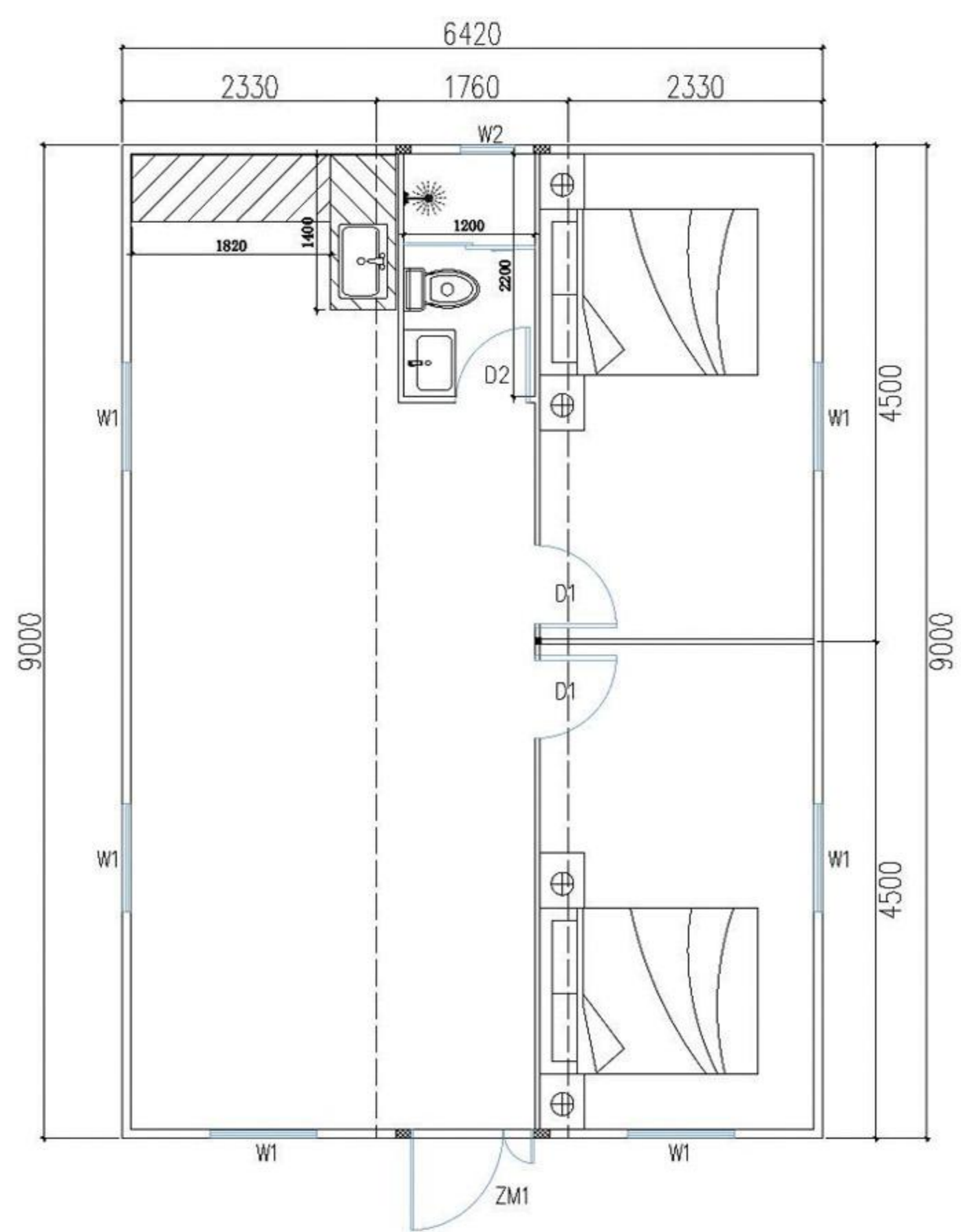
30尺平顶双翼两室一厅一厨一卫平面布置图
