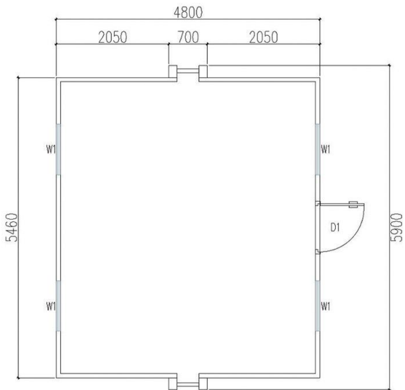
20尺700宽小双翼平面布置图
