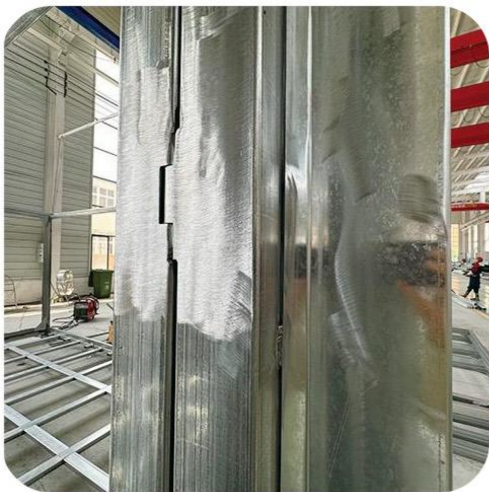
内嵌式合页打磨(Inset hinge sanding)
