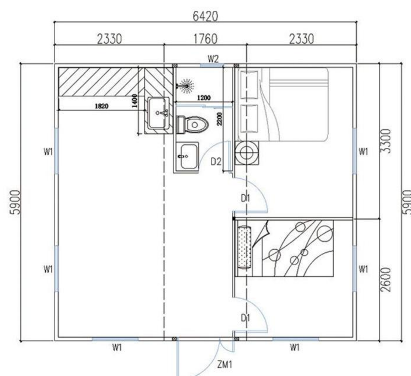
20尺平顶双翼两室一厅一厨一卫平面布置图
