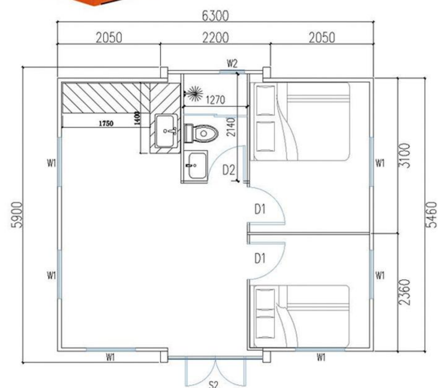
20尺双翼两室一厅一厨一卫平面布置图
