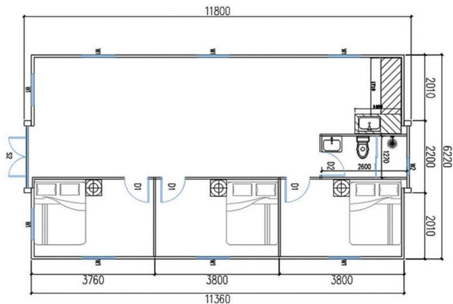
40尺双翼三室一厅一厨一卫平面布置图
