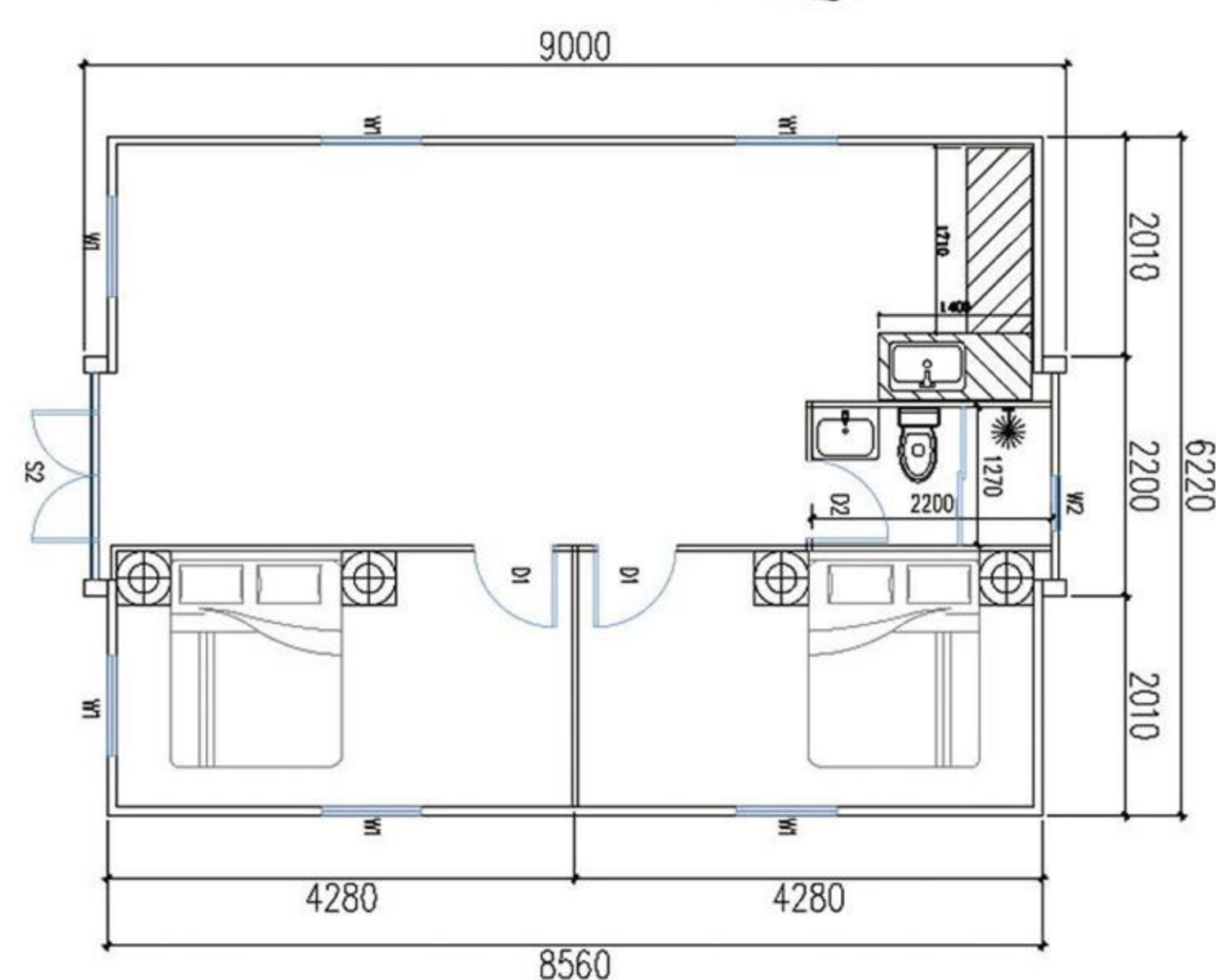
30尺双翼两室一厅一厨一卫平面布置图
